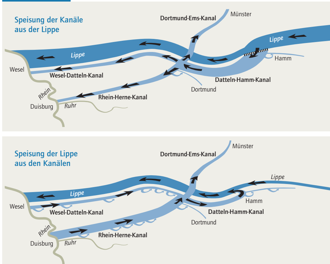
▶ Abb. 3.1.4-2 Schema Wasserüberleitung zur Speisung westdeutscher Kanäle
