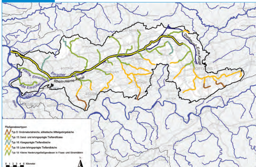
▶ Abb. 2.1.1.1-1 Fließgewässertypen
