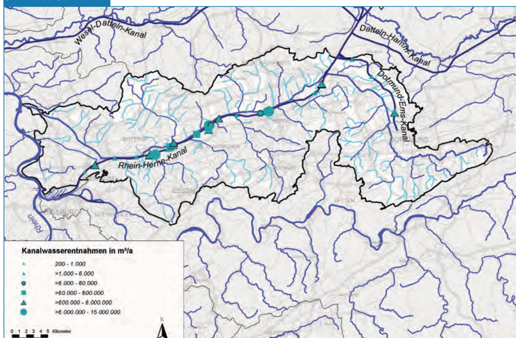
▶ Abb. 3.1.4-1 Erlaubte Wasserentnahmen aus den Schifffahrtskanälen
