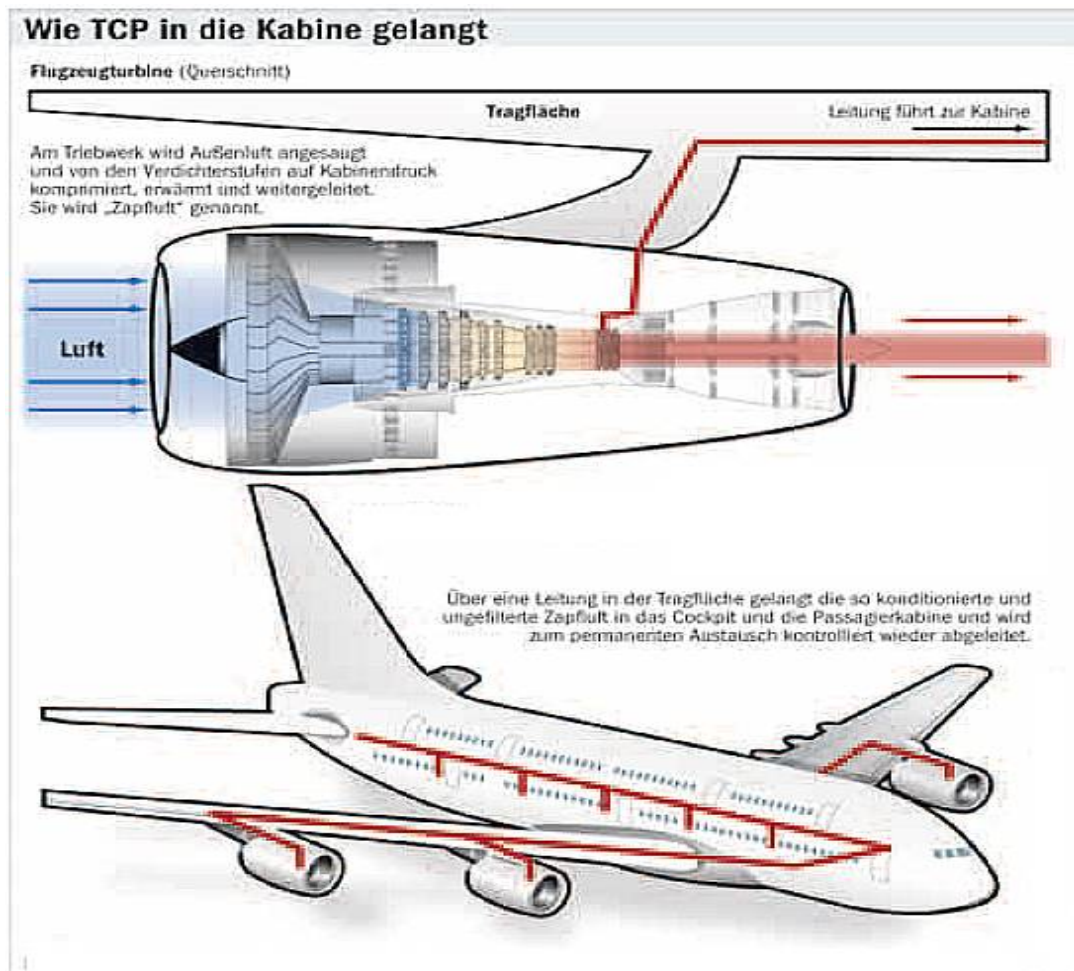
Abb. 1: Triebwerk / Bleed Air (simplifiziert)
