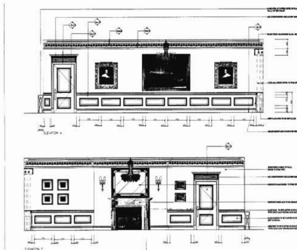
Чертеж гостиной
